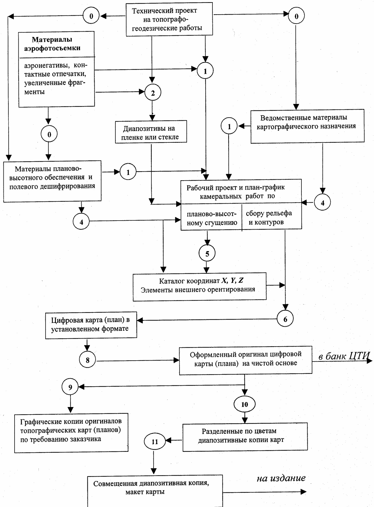
Рис. 1. Технологическая схема камеральных работ при создании цифровых топокарт и планов в масштабах 1:500 - 1:25000 на аналитических фотограмметрических приборах
