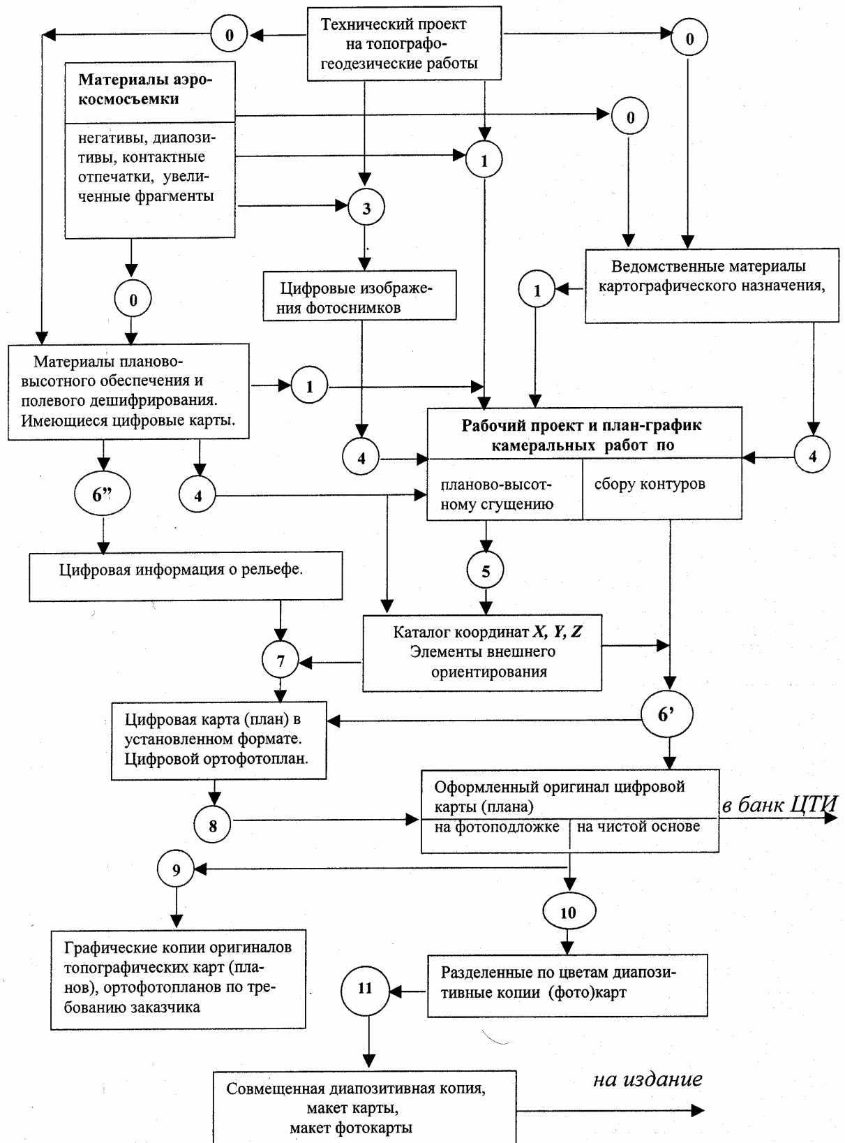
Рис. 3. Технологическая схема камеральных работ при создании цифровых топокарт в масштабах 1:10000 - 1:25000 на цифровых фотограмметрических приборах по одиночным аэрокосмическим снимкам
