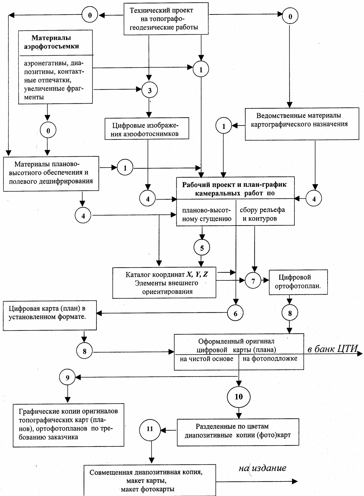
Рис. 2. Технологическая схема камеральных работ при создании цифровых топокарт и планов в масштабах 1:500 - 1:25000 на цифровых фотограмметрических приборах по стереоснимкам
